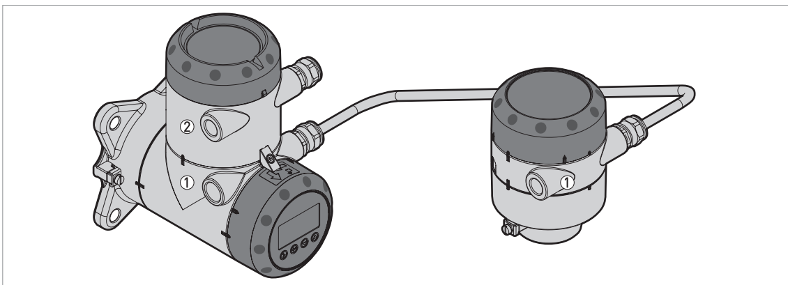
图 3-8：分体（现场）型：腔体属于 Ex d ia 认证的设备
