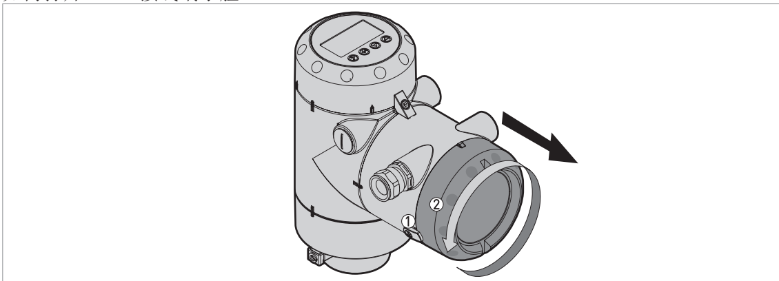
图 3-2：如何打开 Ex d 接线端子腔
