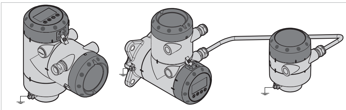
图 3-4: Ex d 应用：端子用于等电位连接系统
