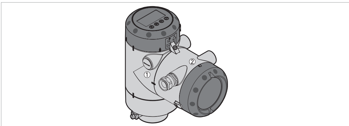
图 3-7：一体型：腔体属于 Ex d ia 认证的设备
